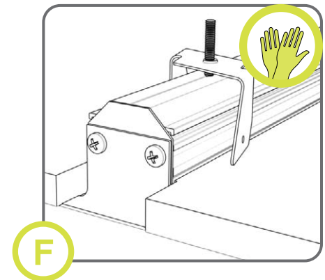
F Repeat step A in reverse to reinstall reflectors, clean top and bottom of lens and reinstall. Répétez l'étape A pour réinstaller le réflecteur et la lentille.
