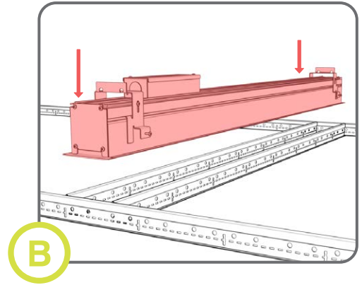
Place fixture in the t-bar ceiling. Placez le luminaire sur la structure du plafond suspendu.
