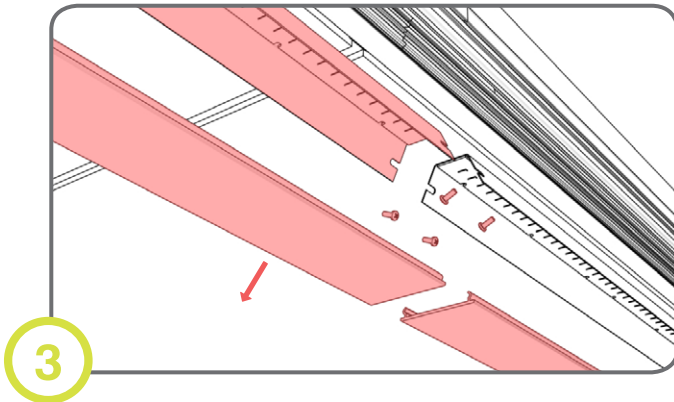
Remove lens, screws and reflector. Enlevez la lentille, les vis et le réflecteur.
