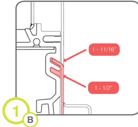
Slot bracket into desired height. Alignez dans l'extrusion.
