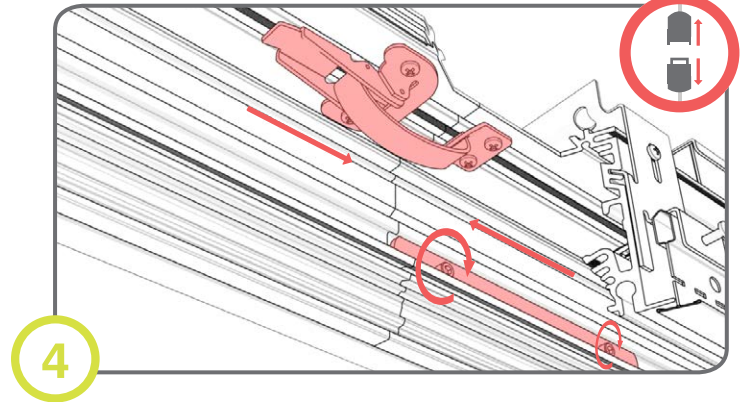
Slide aligning bar into grooves in both sections and secure it with screws. Make connections if required. Faites glisser la barre d'alignement dans les rainures sur les deux sections et serrez les vis. Connectez les câbles si nécessaire.
