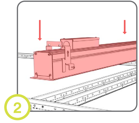
Place fixture sections in the t-bar ceiling. Placez les sections du luminaire sur la structure du plafond suspendu.
